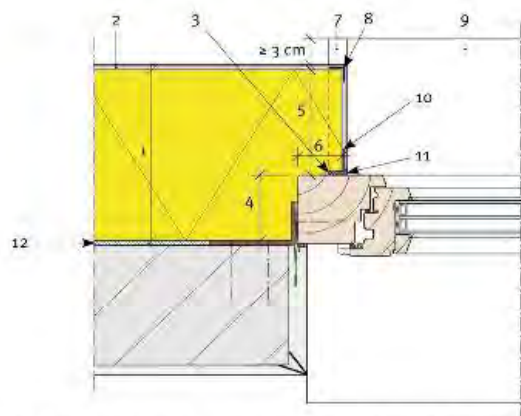
A. Horizontale doorsnede - chassis zonder voorframe (alleen in een geluidsarme omgeving)
