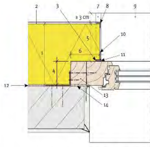
B. Coupe horizontale – Châssis avec précadre
