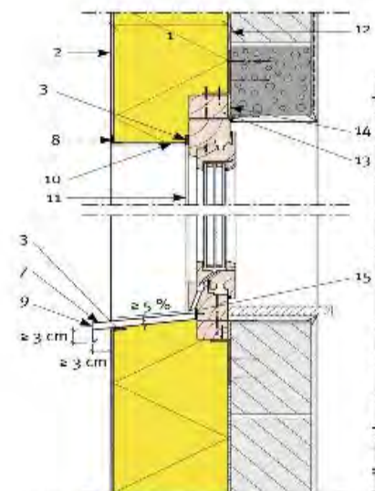
D. Coupe verticale – Châssis avec précadre
