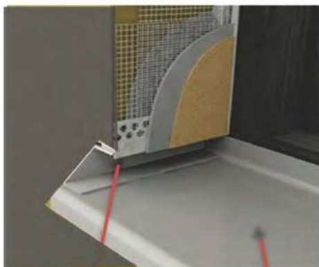
Cornière LX-SPP Pour réhausse latérale des seuils
