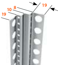
Inneckputzprofil
