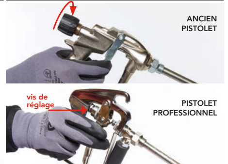
Tourner la vis de réglage et appuyer sur la gâchette pour obtenir un motif de pulvérisation uniforme. A l'aide de la vis de réglage du pistolet professionnel, la largeur de pulvérisation peut être ajustée (voir plus loin).
